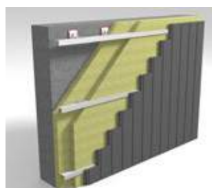
PREFA Siding (vertikálny)
