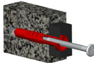
Natĺkanie v plnom tvrdom materiáli
