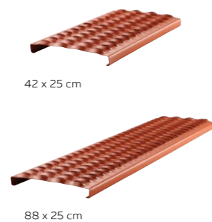
Stúpacia plošina
