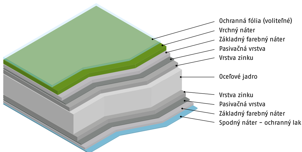
Prierez plechu
