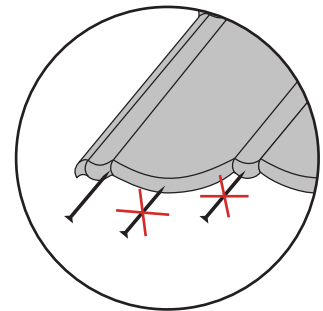
Detail 3.: Detail presného umiestnenia nastreňovacieho klinca do čela panelu.
