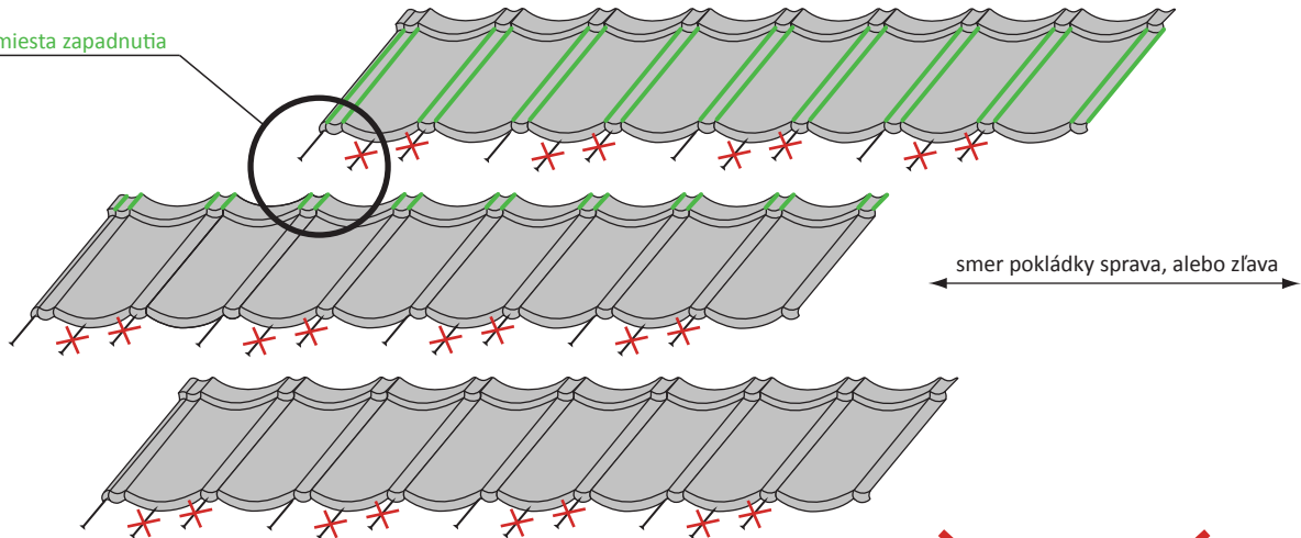
Schéma 1.: Šachovnicové ukladanie panelov v radoch.
