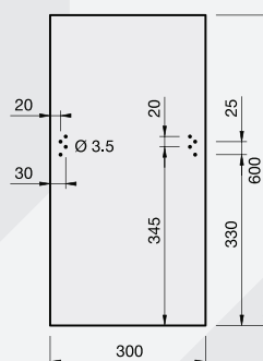
ŠABLÓNA OBDĹŽNIK 30×60 cm
