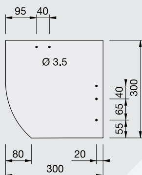
ŠABLÓNA ŠTVOREC S OBLÚKOM 30×30 cm (německé krytí)
