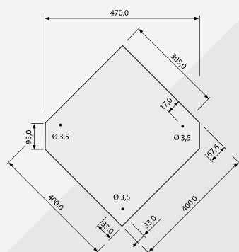
ŠABLÓNA 40×40 cm
