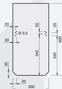
ŠABLÓNA OBDĹŽNIK S KOSEÝMI ROHMI 30×60 cm
