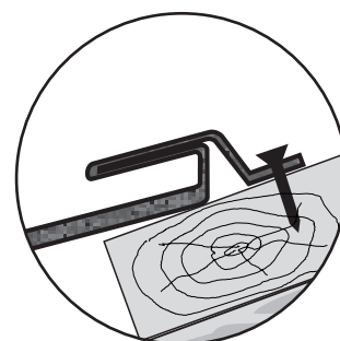
Detail 3.: Detail umiestnenia nastreňovacích klinčov, alebo skrutiek do pásnice sedla panelu
